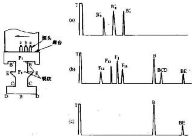
图 A6 双 T 型叶根检验时动态波形过程图
