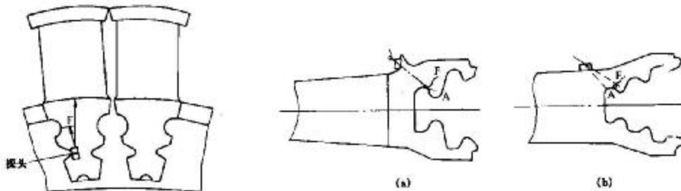
(a) 带汽封菌形叶根检验；(b) 不带汽封菌形叶根检验 图8 菌形叶根检验时探头放置图
